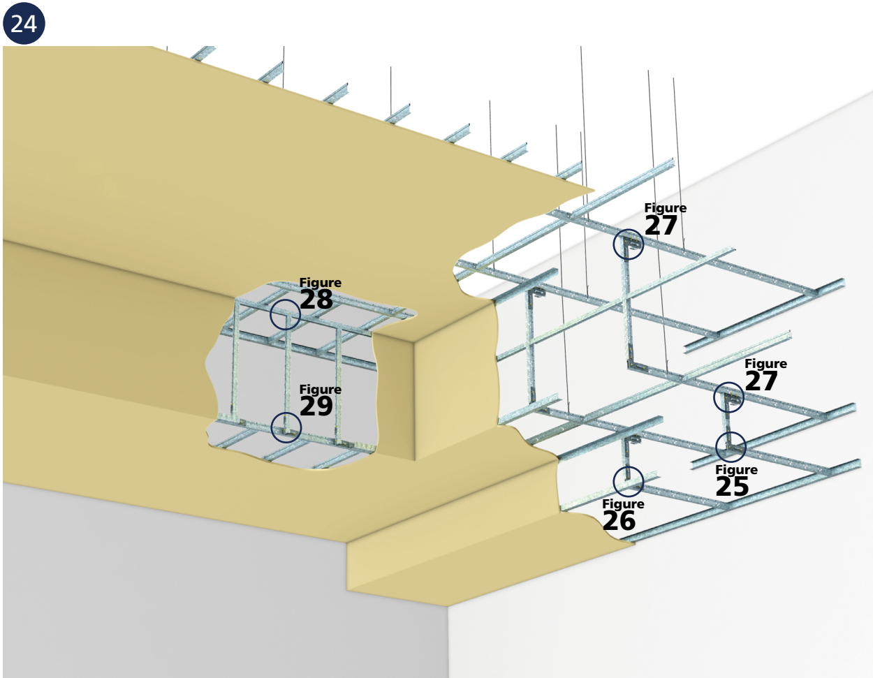
■ RONDO XPRESS® DRYWALL GRID BULKHEAD/SOFFIT
